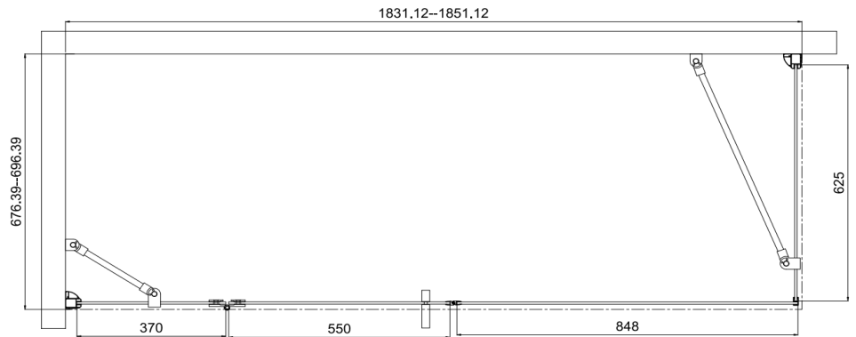
Esempio Porta battente 100 + In-Line 90 + Lato fisso 70
