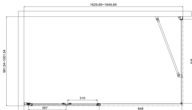
Esempio Porta pieghevole 80 + In-Line 90 + lato fisso 80
