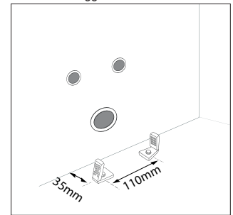
Schema fissaggio a terra
