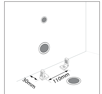
Schema fissaggio a terra
